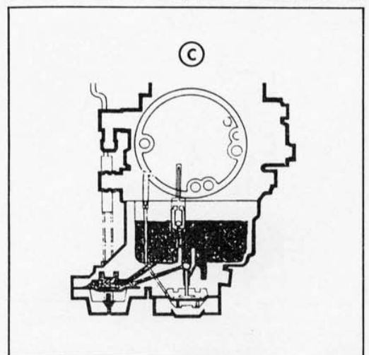
A) Motore spento scarico pompa / Engine off pump discharge B) Motore acceso scarico pompa / Engine on pump discharge C) Motore acceso aspirazione pompa / Engine on pump intake 1) Sfera in sede / Ball seated 2) Sfera non in sede / Ball unseated
