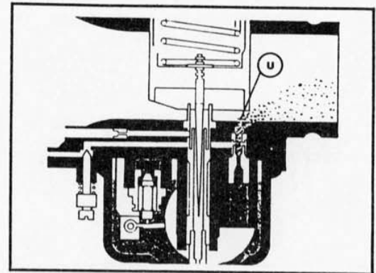
u) Circuito di transizione / Transition circuit
