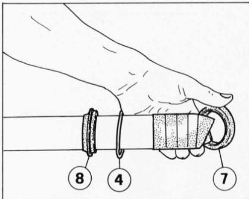
4) Fermo raschiaolio / Ring oil seal stop / L'arrêt raclleur d'huile / Ölabbstreifer / Tope raspa-aceite 7) Raschiaolio / Oil seal / Pare-huile / Ölabdichtung / Tope raspa-aceite 8) Parapolvere / Dust seal / Pare-poussière / Pulverdeckel / Placa retención polvo
