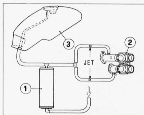
1) Cannister 2) Carburatore 3) Serbatoio del carburante
